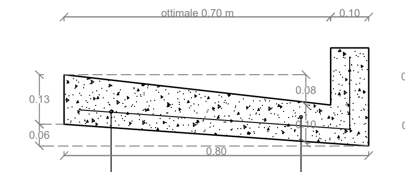
BANCHINA/CUNETTA IN CLS TIPO B 1:10
