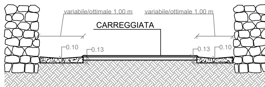
SEZIONE TIPO IN PROGETTO - BANCHINA/CUNETTA IN CLS TIPO A 1:50
