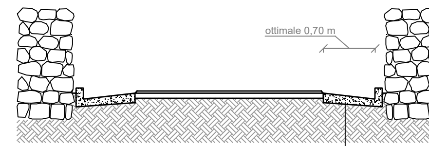
SEZIONE TIPO IN PROGETTO - CUNETTA IN CLS TIPO B 1:50
