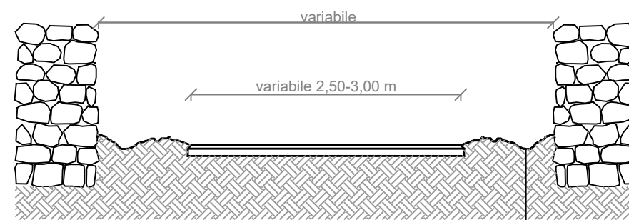
SEZIONE TIPO - SITUAZIONE ESISTENTE 1:50
