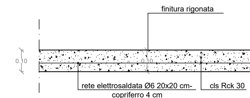
SEZIONE TIPO PAVIMENTAZIONE STRADALE IN CLS 1:10
