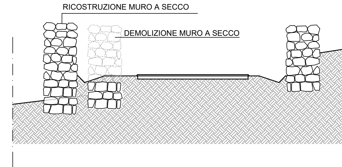
SEZIONE TIPO IN PROGETTO - DEMOLIZIONE /RICOSTRUZIONE MURI 1:50
