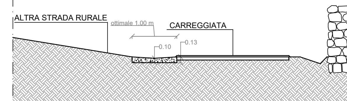
SEZIONE TIPO IN PROGETTO - INCROCI CON ALTRE STRADE BANCHINA/CUNETTA IN CLS TIPO A 1:50
