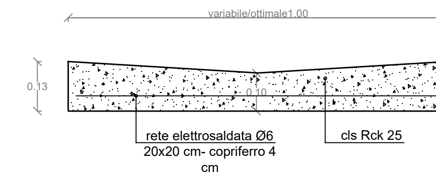
BANCHINA/CUNETTA IN CLS TIPO A 1:10
