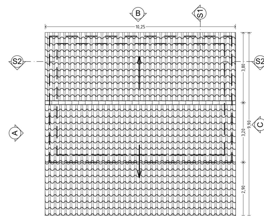
PIANO COPERTURA SCALA 1:100
