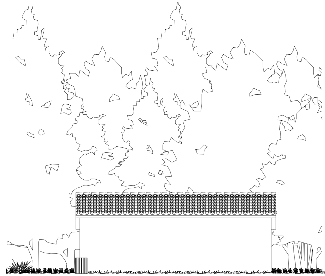
PROSPETTO B SCALA 1:100
