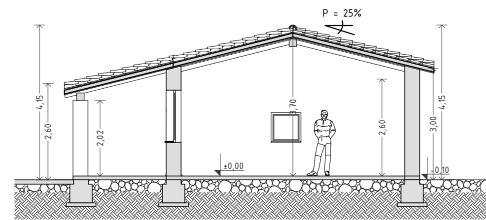
SEZIONE S1 SCALA 1:100
