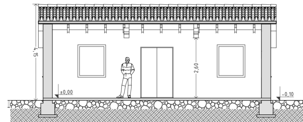
SEZIONE S2 SCALA 1:100
